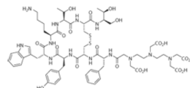
DTPA-TOC trifluoroacetate DTPA-O-Phe-Cys-Tyr-D-Trip-Lys-Thr-Cys-Thr(ol)
