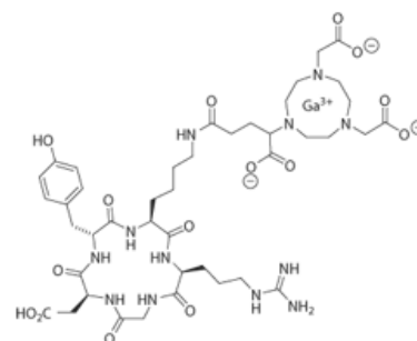
Ga-NODAGA-RGD Arg-Gly-Asp-D-Tyr-Lys[NODAGA(Ga)]
